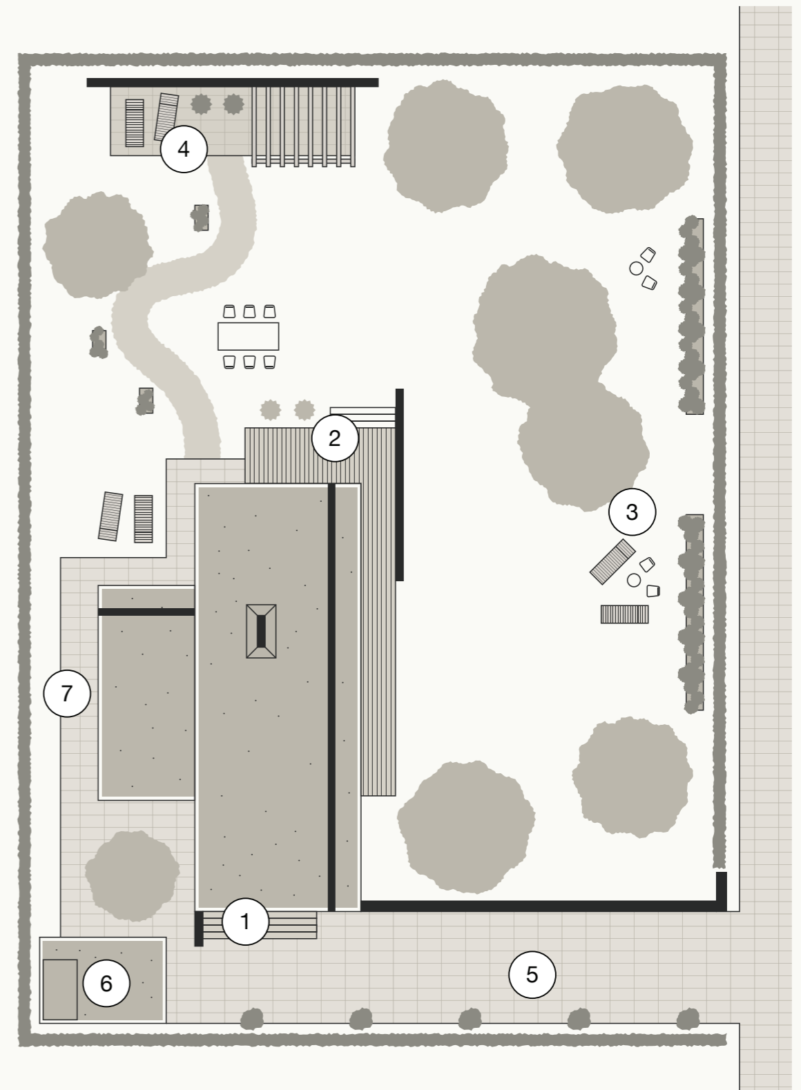
1. Toegang, 2. Dakterras en terras, 3. Garden, 4. Patio en serre, 5. Oprit en pad, 6. Garage, 7. Bewegwijzering
